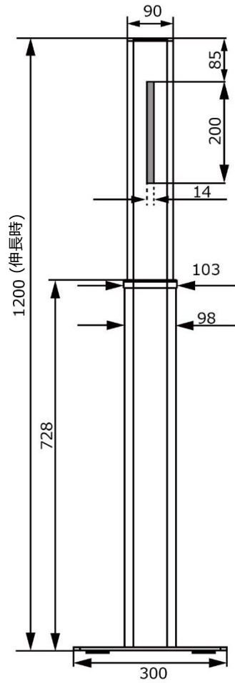
正面図
