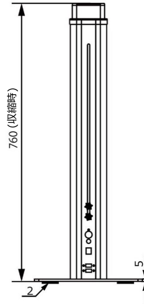
背面図
