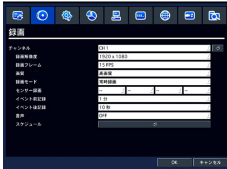
図 録画メニュー画面
