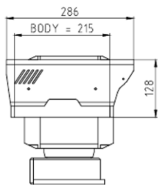
左側面
