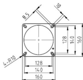
底面
