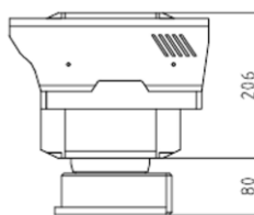
右側面
