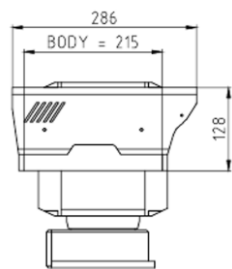
左側面
