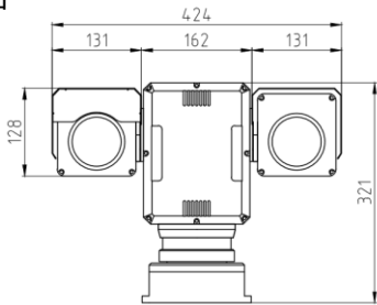
正面
